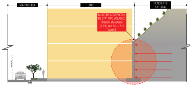
Imagen N° 4: muro de contención en terrenos con pendiente
