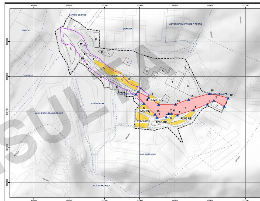
Imagen N° 9: MP-GRD 01 Propuesta de prevención de riesgo no estructural.
