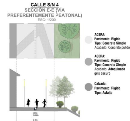
Imagen N° 8: sección de pasaje peatonal de la ZRESA08
