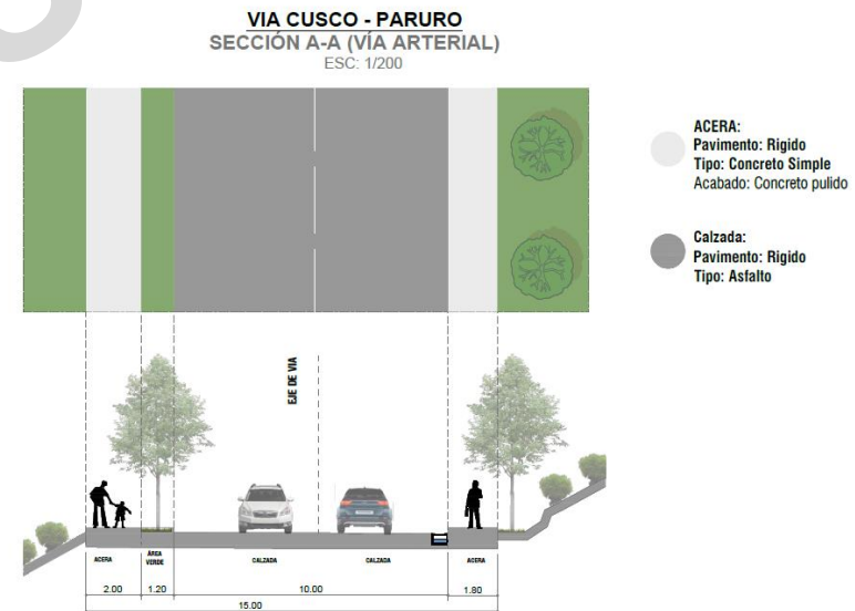
Imagen N° 5: sección de vía arterial de la ZRESA08
