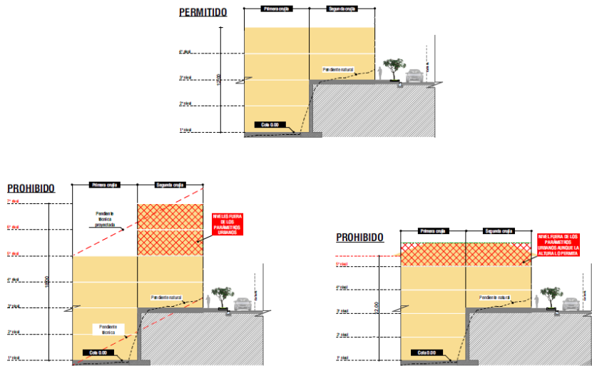
Imagen N° 2: altura edificatoria permitida de lote con lado longitudinal en pendiente
