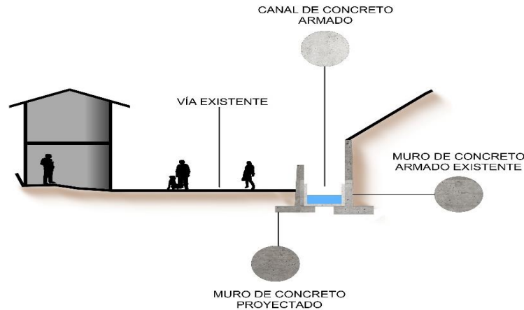
Imagen N°71: Muro de contención.
